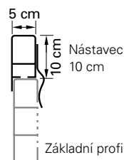
Dvoudílný základní profil
