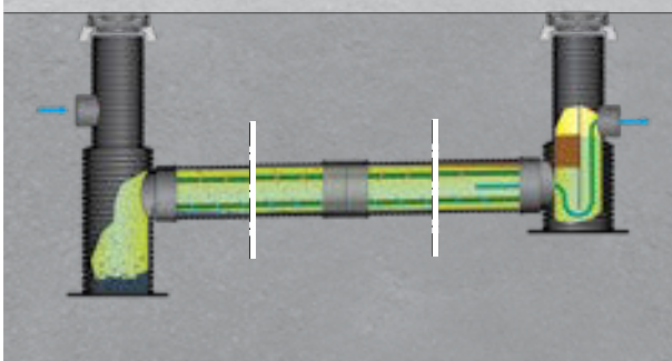
SediPipe – sedimentační zařízení se sedimentační trubkou
