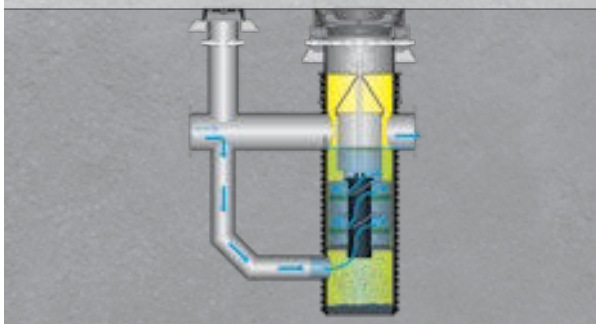
SediSubstrator – sedimentační zařízení se sedimentační trubkou a substrátovým stupněm
